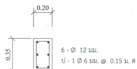
แบบขยายรูปตัดคาน 1 : 25
