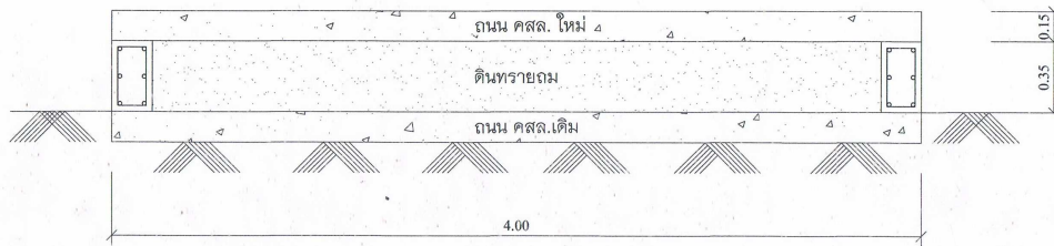
แบบขยายรูปตัดถนน 1 : 25
